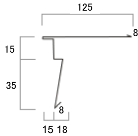
スパンルーフ 改修用唐草
